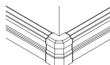
＜出隅役物納まり図＞
